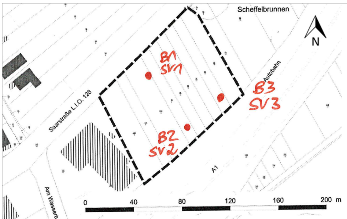
Abbildung 6: Lageplan des ursprünglichen Gebietes mit Untersuchungsstellen
