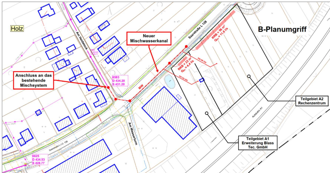
Abbildung 9: Entwässerungskonzept
