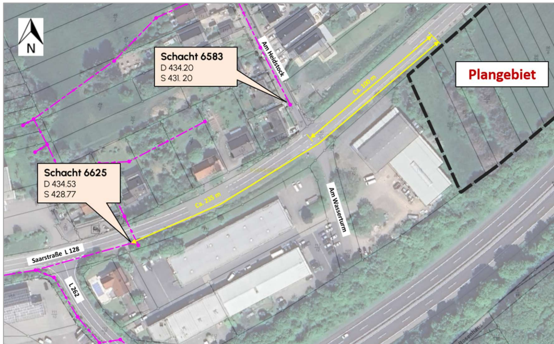
Abbildung 5: Bestehende Anlagen der Siedlungsentwässerung
