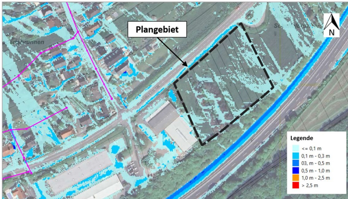
Abbildung 4: Überflutungstiefen infolge Starkregen
