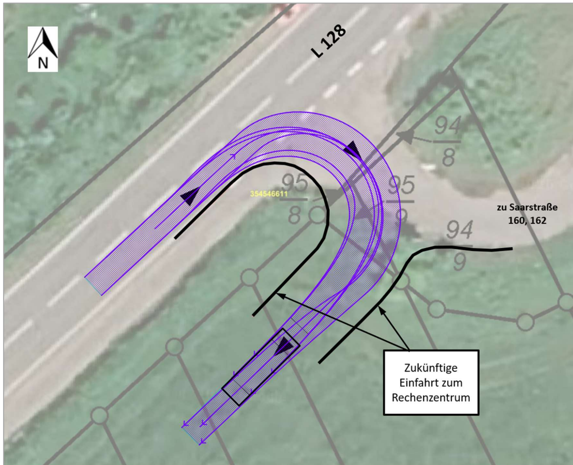
Abbildung 11: Schleppkurvenprüfung für den kritischen Fall eines Rechtsabbiegers aus Richtung Holz kommend
